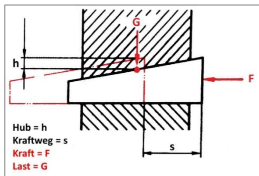
Abbildung 17: Keilwirkung (U. Fischer et al., 1990, S. 131)
