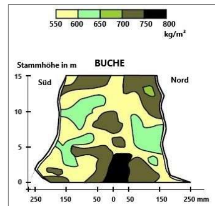
Abbildung 32: Darstellung der Inhomogenität einer Buche (Thienel, 2016, S. 23)
