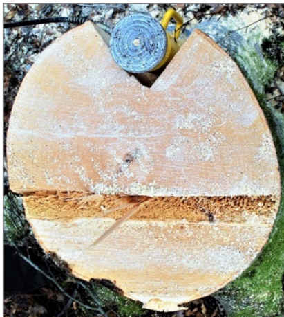
Abbildung 67: Abbild eines Stocks mit Hubzylinder nach dem Fällen (Eigene Darstellung)
