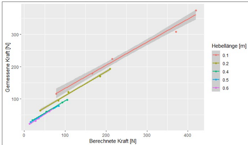
Abbildung 76: Verhältnis von gemessener zu berechneter Kraft unter Einfluss der Hebellänge (Eigene Darstellung)
