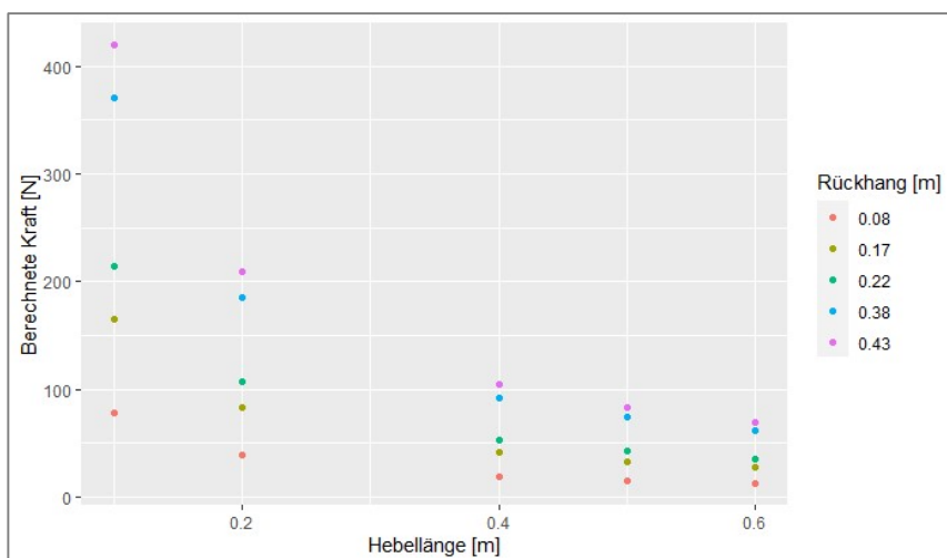
Abbildung 71: Berechnete Kraft in Abhängigkeit von der Hebellänge (Eigene Darstellung)
