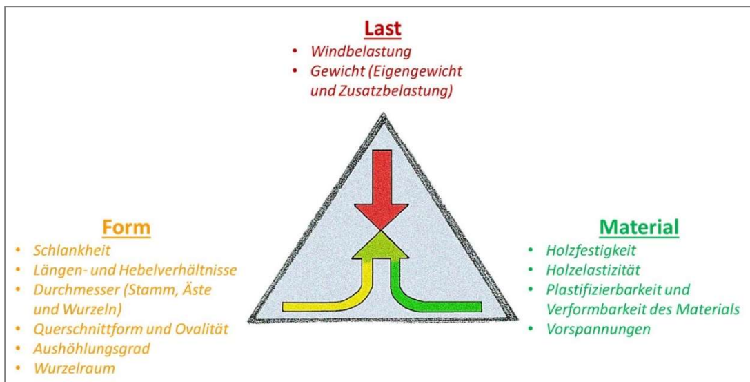
Abbildung 6: Dreieck der Statik am Baum (Wessolly & Erb, 2014, S. 94)
