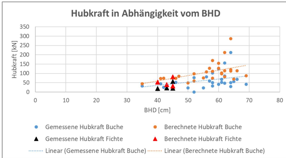
Abbildung 101: Hubkraft in Abhängigkeit vom BHD (Eigene Darstellung)
