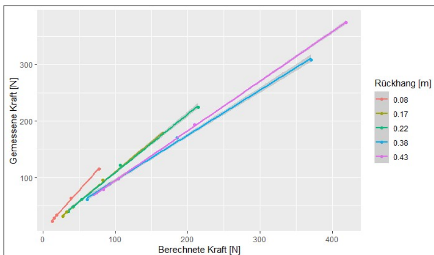
Abbildung 77: Verhältnis von gemessener zu berechneter Kraft unter Einfluss des Rückhangs (Eigene Darstellung)
