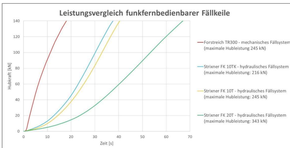
Abbildung 22: Leistungsvergleich mechanischer und hydraulischer Funkfernkeile (Ruppert & Lippert, 2019a)
