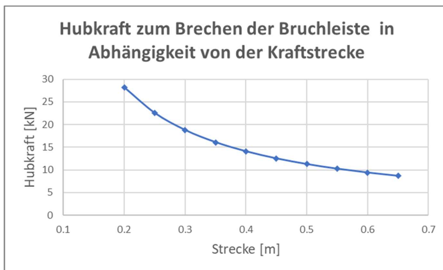
Abbildung 83: Hubkraft zum Brechen der Bruchleiste in Abhängigkeit von der Strecke zwischen Drehpunkt und Kraftangriffspunkt (Eigene Darstellung)
