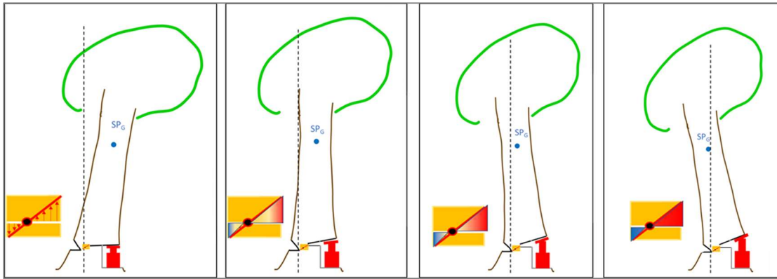
Abbildung 79: Darstellung der Beanspruchung der Bruchleiste (Eigene Darstellung)
