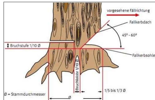
Abbildung 25: Stockmaße bei der Baumfällung (DGUV 2011)
