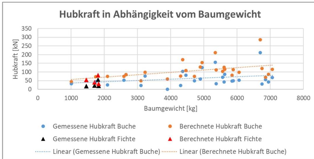
Abbildung 102: Hubkraft in Abhängigkeit vom Baumgewicht (Eigene Darstellung)
