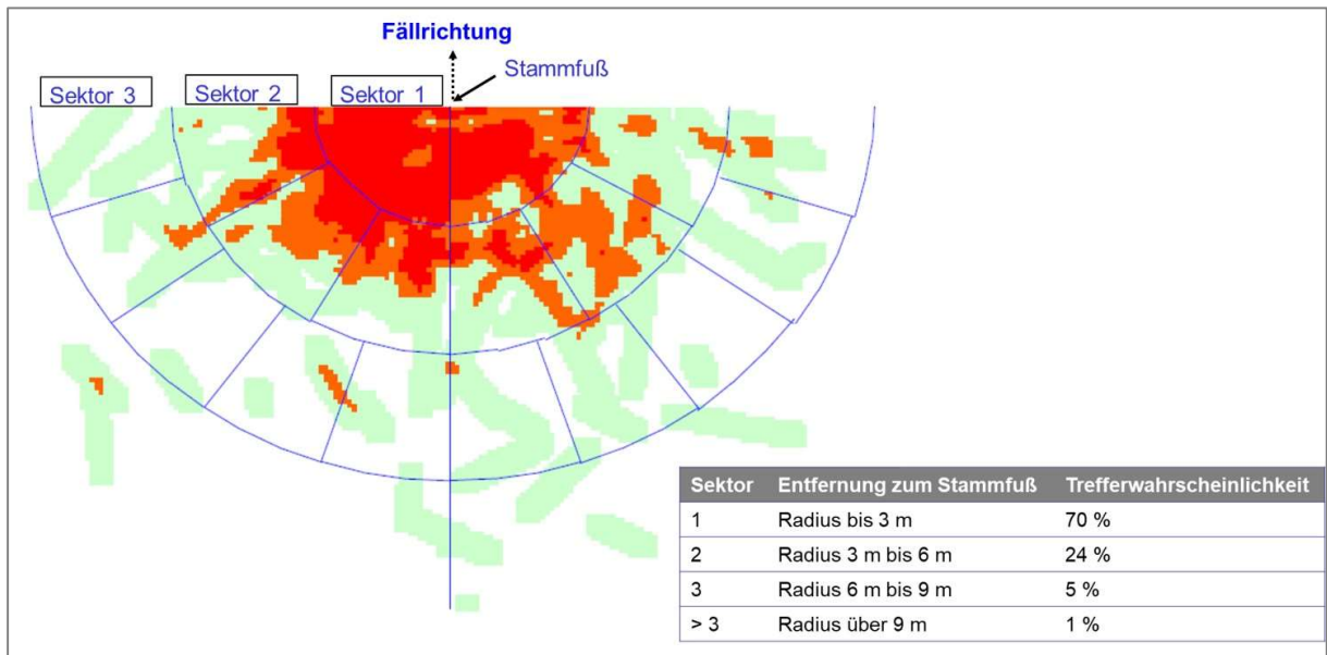
Abbildung 3: Wahrscheinlichkeit eines Asttreffers in Abhängigkeit von der Entfernung zum Stock (Gerding & Reiter, 2010)
