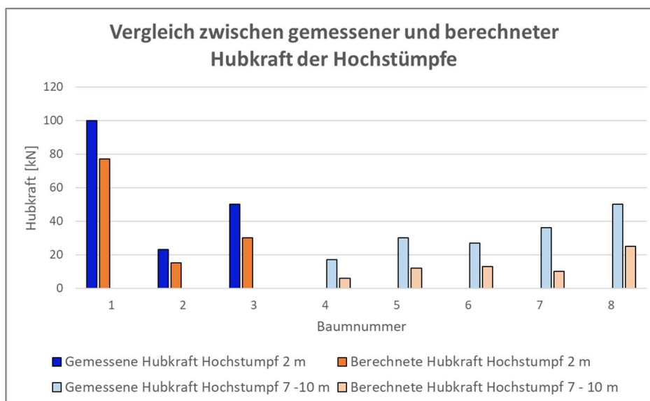
Abbildung 89: Vergleich zwischen gemessener und berechneter Hubkraft der Hochstümpfe (Eigene Darstellung)
