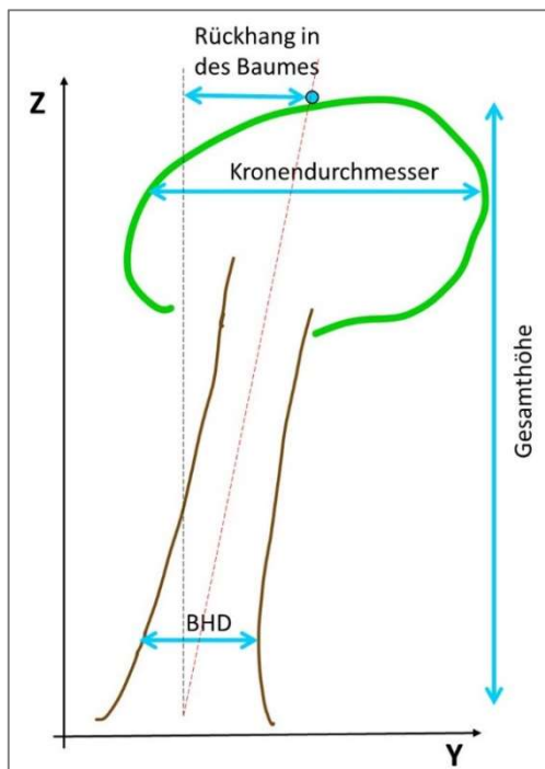
Abbildung 103: Skizze für die Hubkraftkalkulation (Eigene Darstellung)
