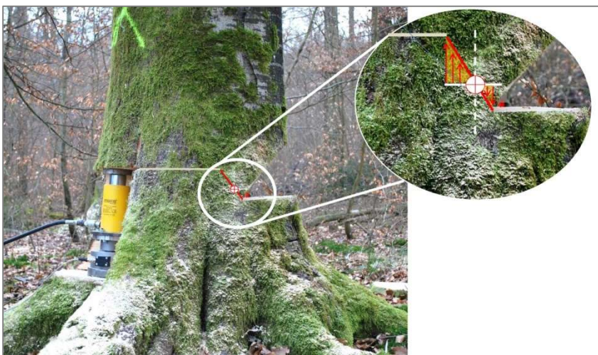
Abbildung 9: Darstellung der Biegespannung in der Bruchleiste (Eigene Darstellung)
