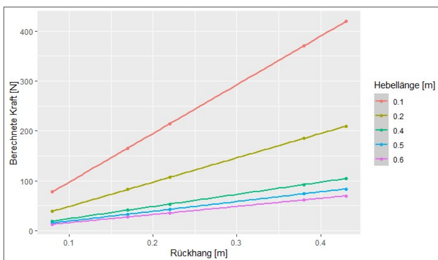
Abbildung 70: Berechnete Kraft in Abhängigkeit vom Rückhang (Eigene Darstellung)
