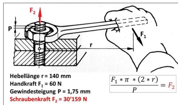
Abbildung 18: Schraubenkraft am Gewinde (U. Fischer et al., 1990, S. 132)
