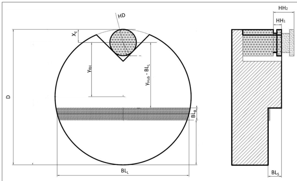
Abbildung 68: Zeichnung eines Stockbildes inkl. Hubzylinder (Eigene Darstellung)
