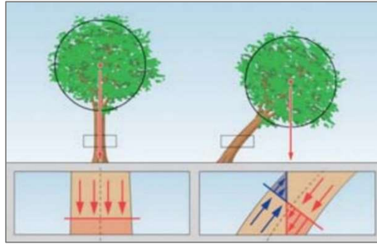
Abbildung 8: Biegemomente bei schrägstehenden Bäumen (deritec GmbH)
