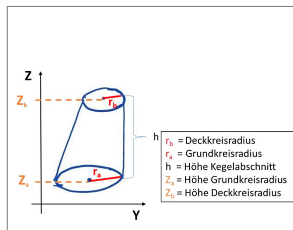
Abbildung 52: Einzelansichtsskizze eines Kegelstumpfs (Eigene Darstellung)
