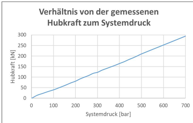
Abbildung 64: Verhältnis von der gemessenen Hubkraft zum Systemdruck (Eigene Darstellung)
