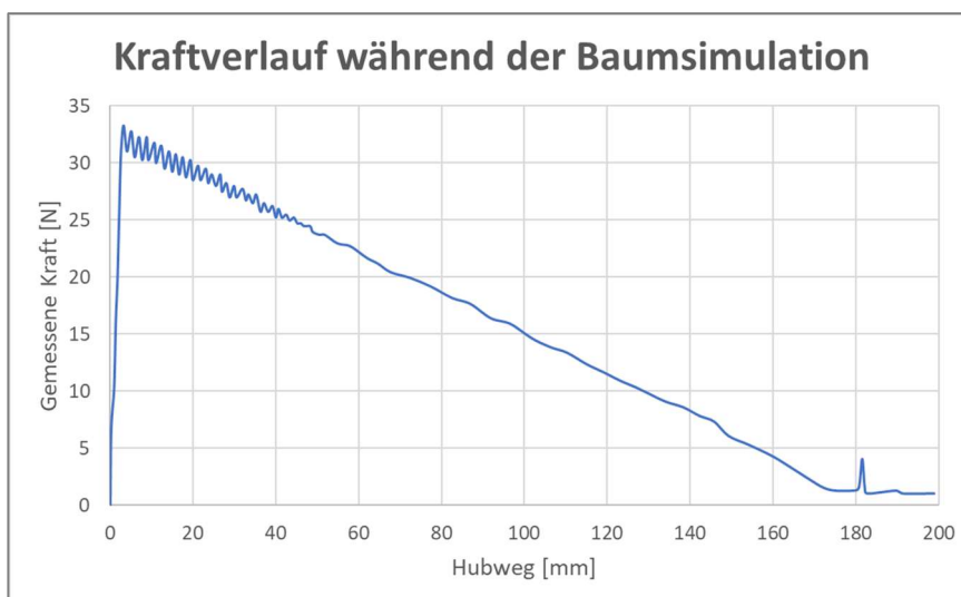
Abbildung 72: Kraftverlauf während der Schwerpunktverlagerung (Eigene Darstellung)
