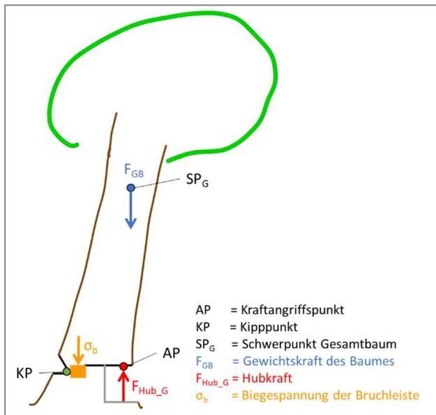
Abbildung 33: Freischnitt der Kräfte und Spannungen während der Baumfällung mit einer Fällhilfe (Eigene Darstellung)
