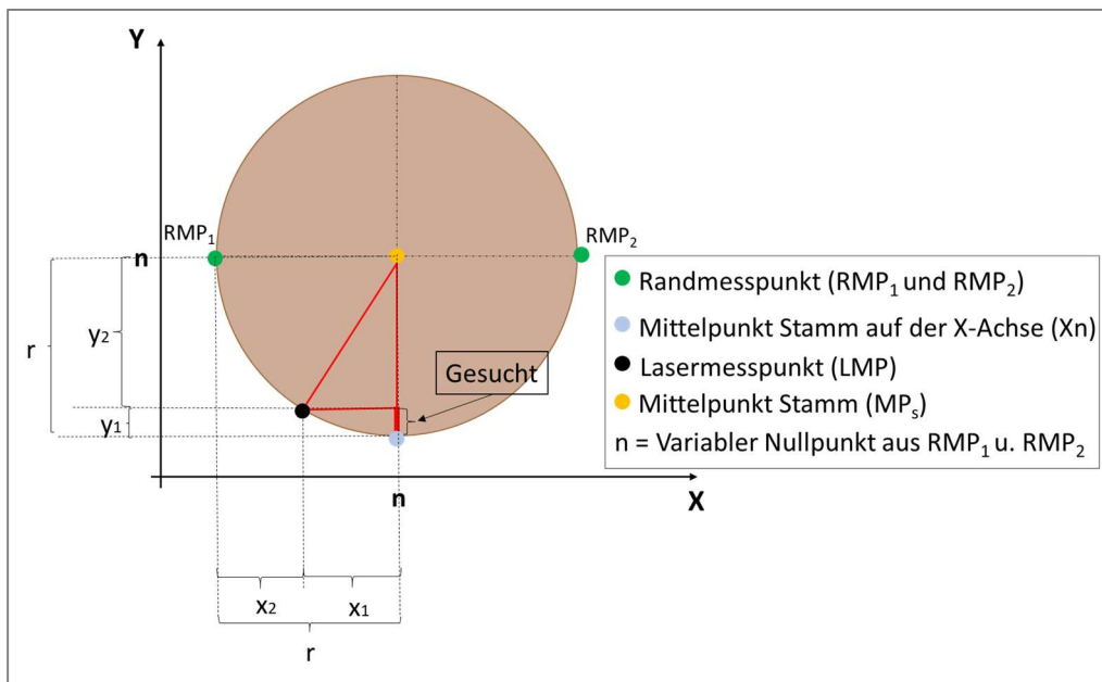
Abbildung 44: Skizze der Korrektur der Lasermessdaten hinsichtlich des Stammdurchmessers (Eigene Darstellung)
