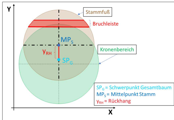
Abbildung 58: Skizze des Baumrückhangs (Draufsicht) (Eigene Darstellung)
