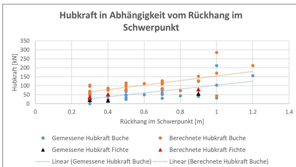
Abbildung 100: Hubkraft in Abhängigkeit vom Rückhang im Schwerpunkt (Eigene Darstellung)
