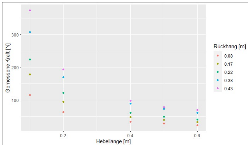
Abbildung 73: Gemessene Kraft in Abhängigkeit von der Hebellänge (Eigene Darstellung)
