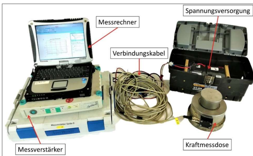
Abbildung 63: Verwendete Messmittel zur Bestimmung der Hubkraft bei der Fällung von Bäumen (Eigene Darstellung)
