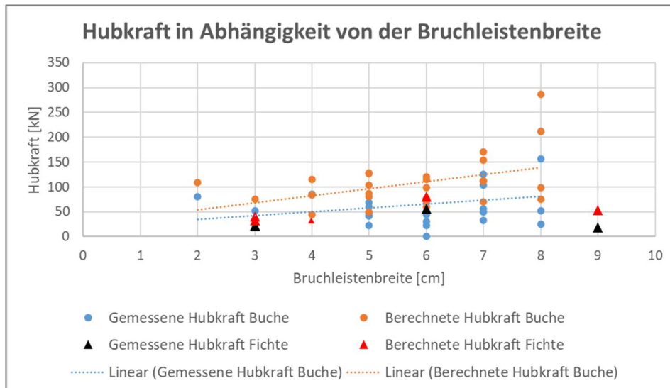
Abbildung 99: Hubkraft in Abhängigkeit von der Bruchleiste
