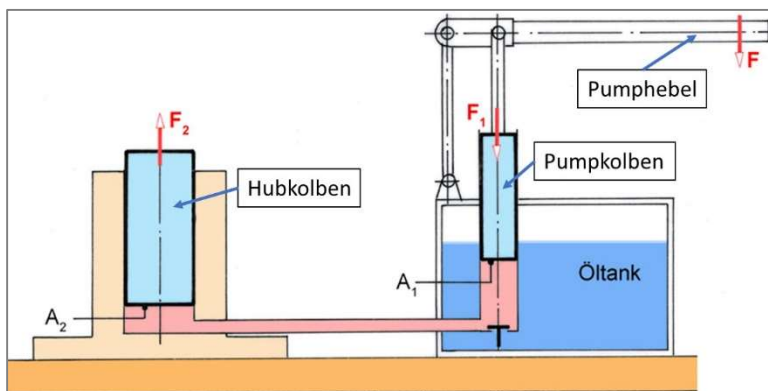
Abbildung 20: Funktionsweise der hydraulischen Presse (lehrerfreund.de, 2010)
