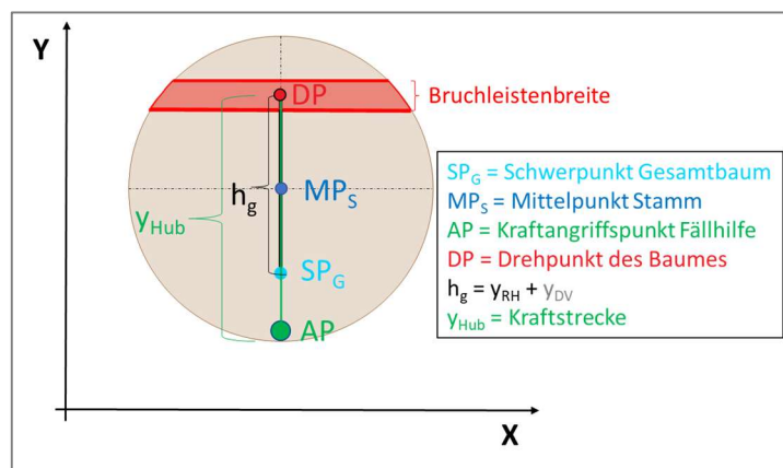
Abbildung 60: Skizze zur Hubkraftermittlung (Draufsicht) (Eigene Darstellung)
