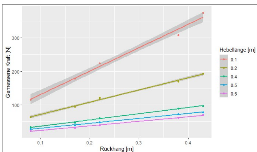
Abbildung 74: Gemessene Kraft in Abhängigkeit vom Rückhang (Eigene Darstellung)
