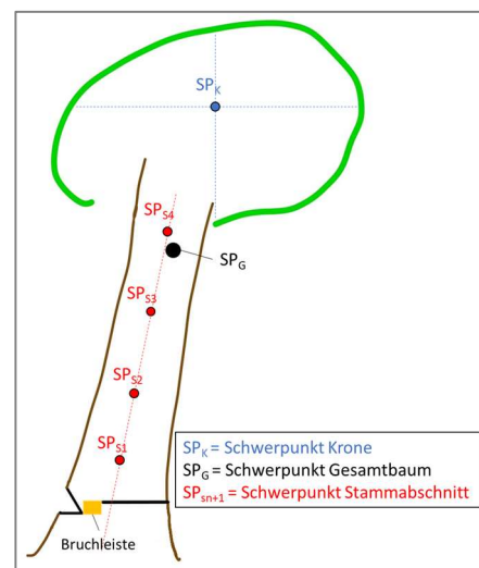
Abbildung 56: Skizze des resultierenden Gesamtschwerpunktes im Baum (Eigene Darstellung)
