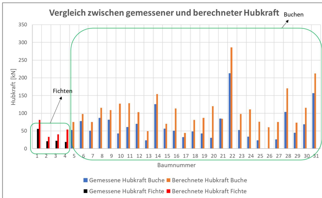
Abbildung 98: Vergleich zwischen gemessener und berechneter Hubkraft (Eigene Darstellung)
